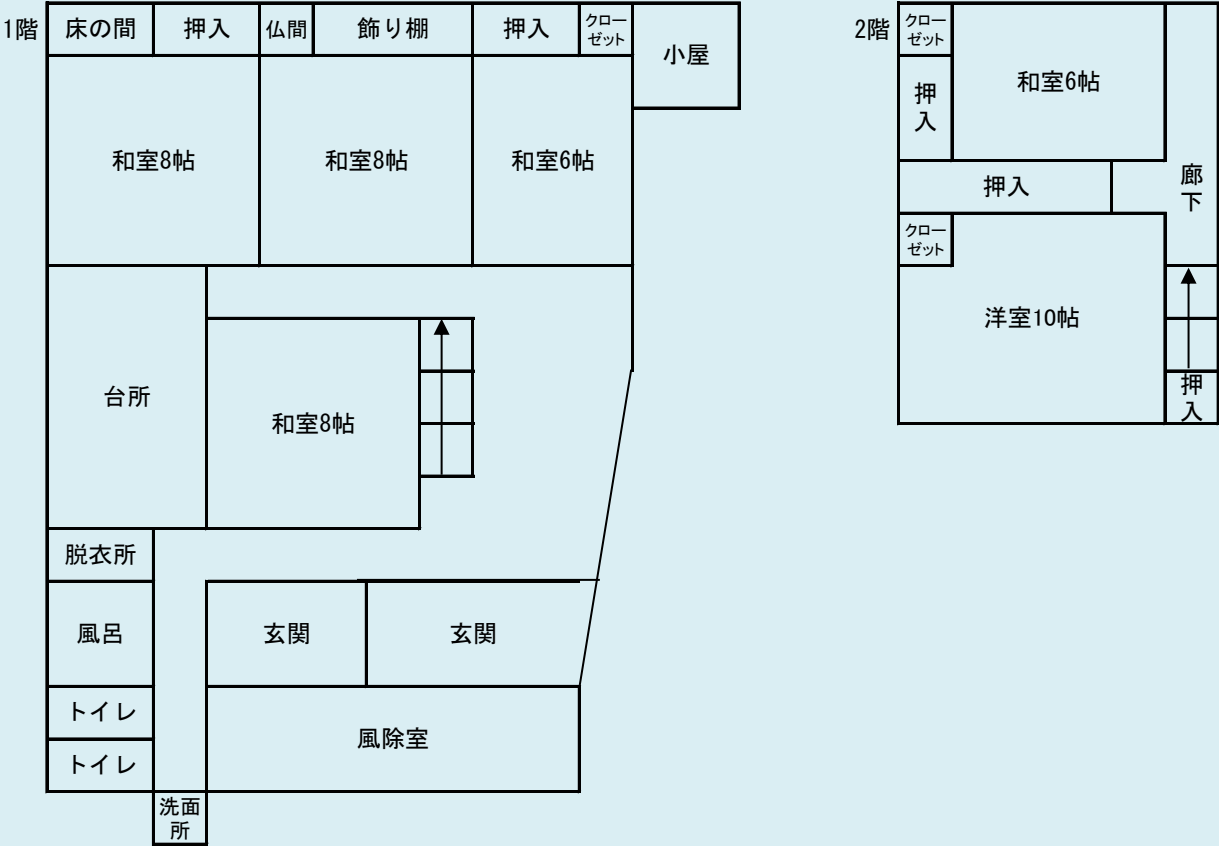
間取り（概況）
