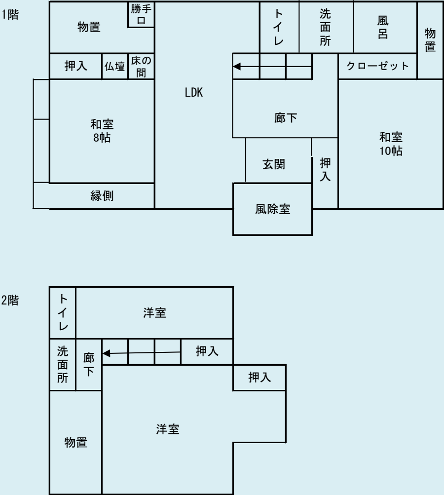
間取り（概況）
