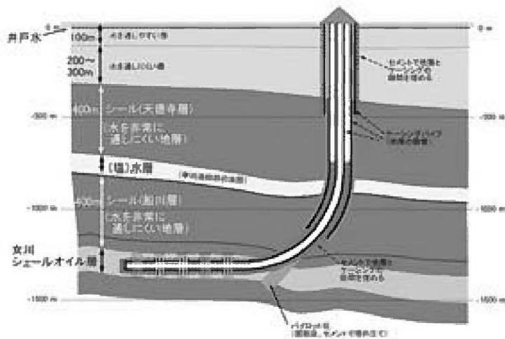
【フラクチャリングの概念図】
