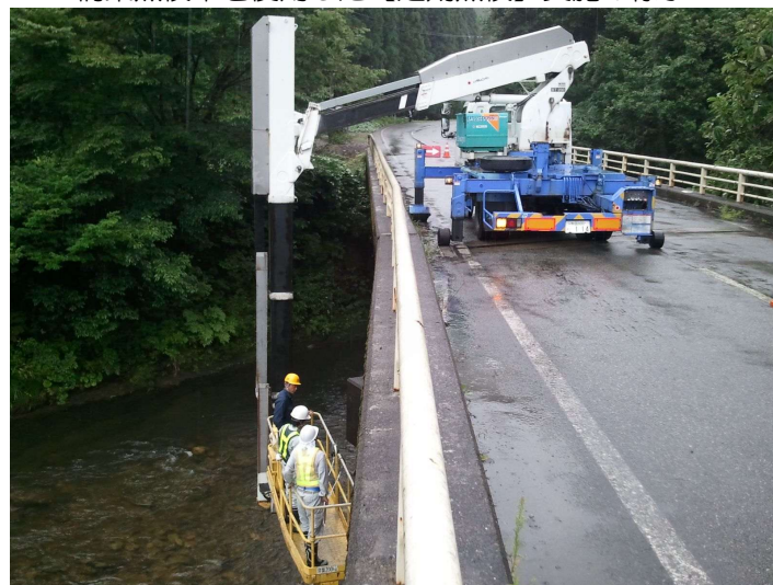
橋梁点検車を使用した【定期点検】実施の様子
